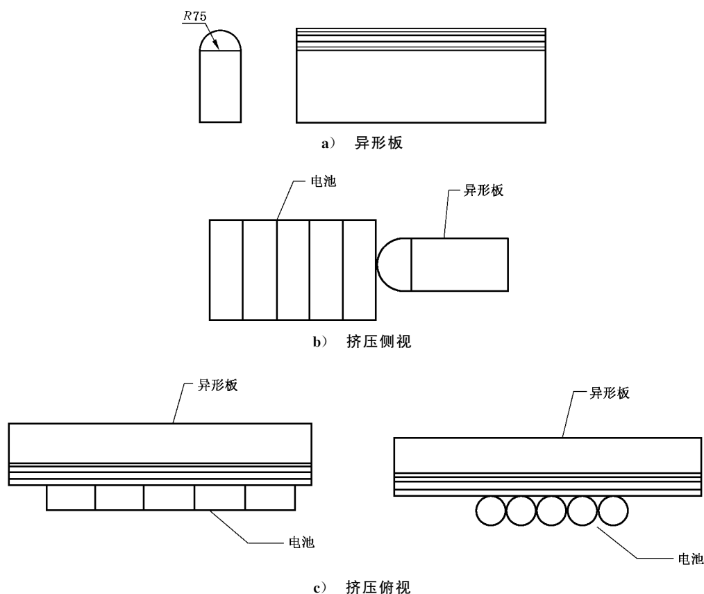
图 1 异形板和挤压示意图
